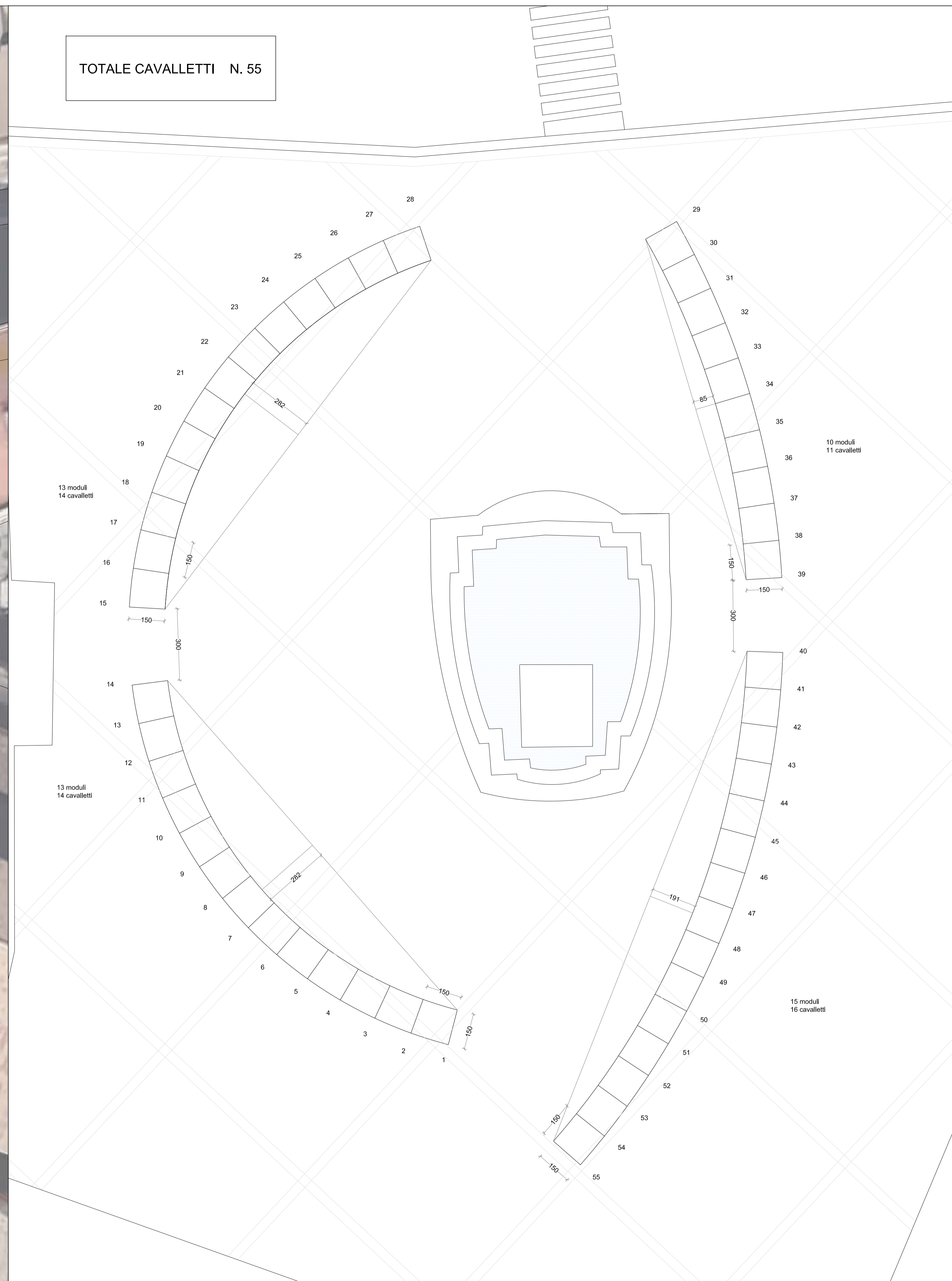
PIANTA 1:100
