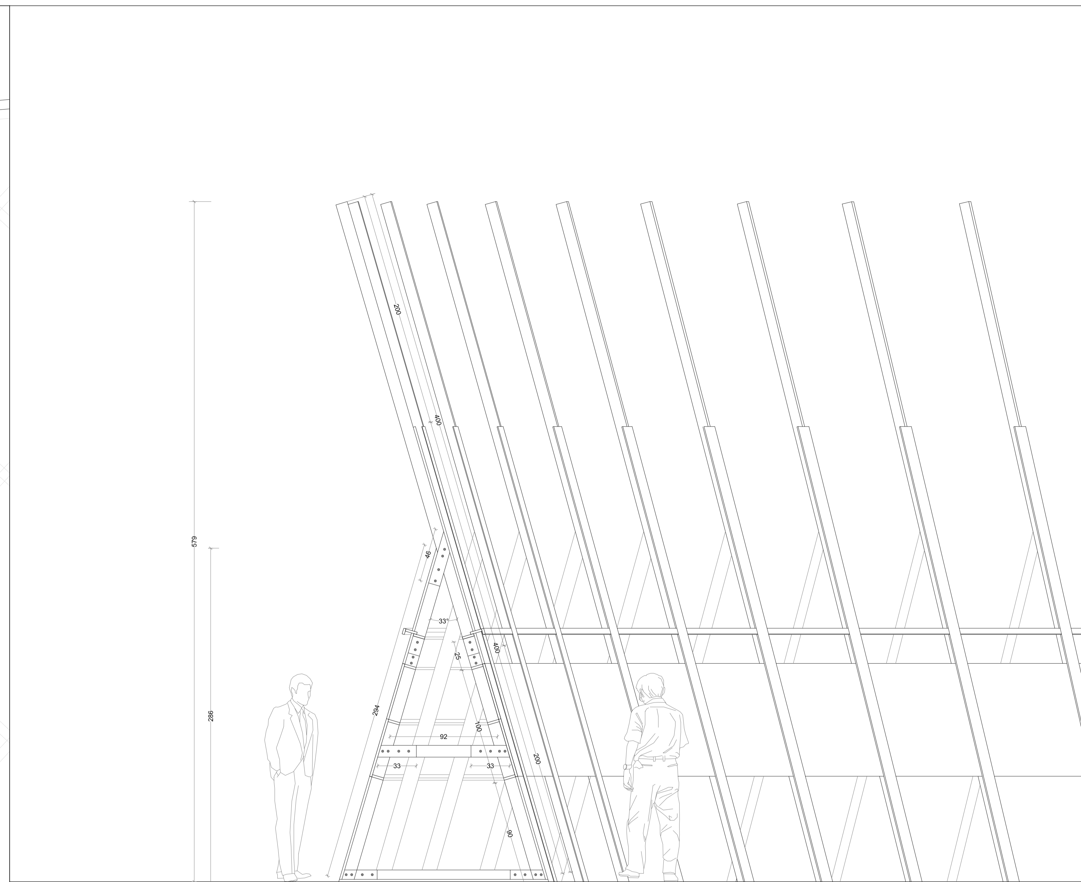
SEZIONE 1:20
